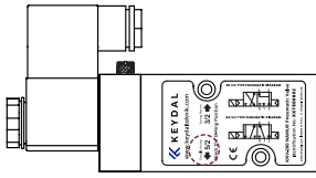
5/2 Tip Ayarlı Solenoid Valf
